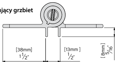
KF3L2 - Boczne wsporniki L2
